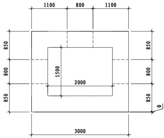
790沉沙池平面图
