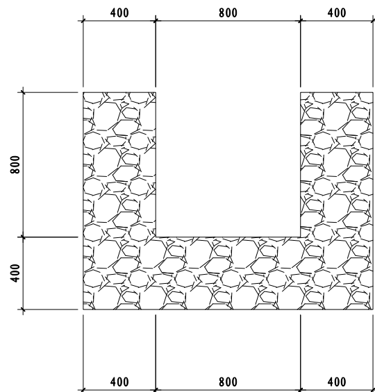
790-830左岸截洪沟剖面图
